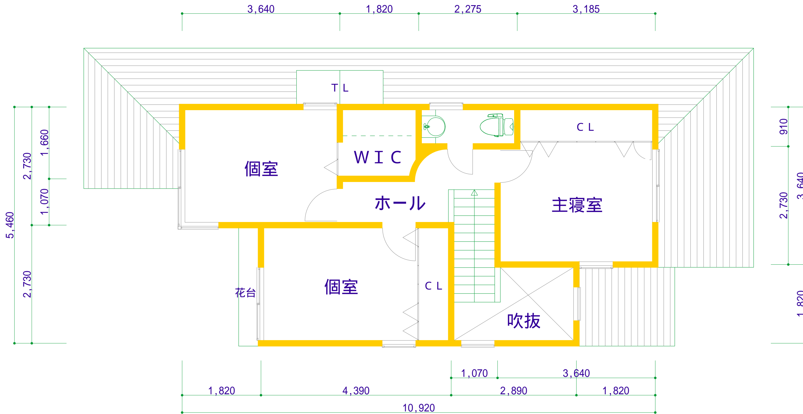
2階平面図
